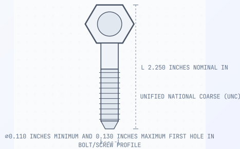
5306-00-059-8649 — BOLTS
